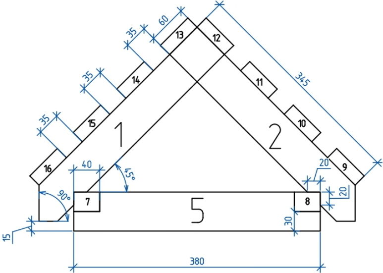
Стропильная система вид спереди
